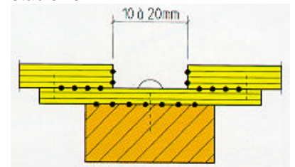
Figuur 4 Verticale naad variant.
