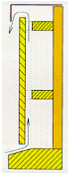
Figuur 5 Schematische voorstelling van de wijze van ventileren.
